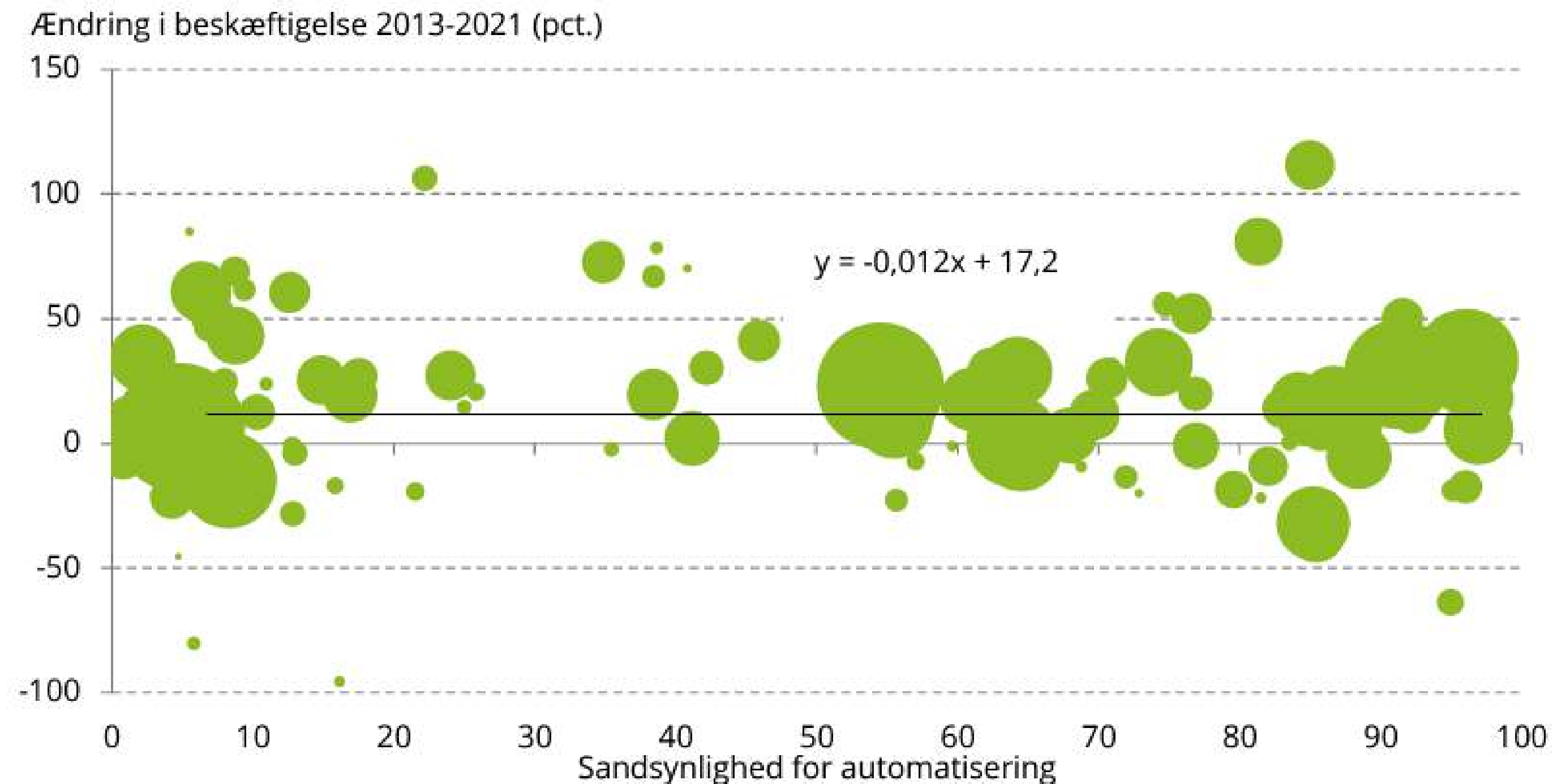
Figur 4.6 Sammenhæng mellem automatiseringssandsynlighed i 2013 og beskæftigelsesudviklingen fra 2013 til 2021 på tværs af job
